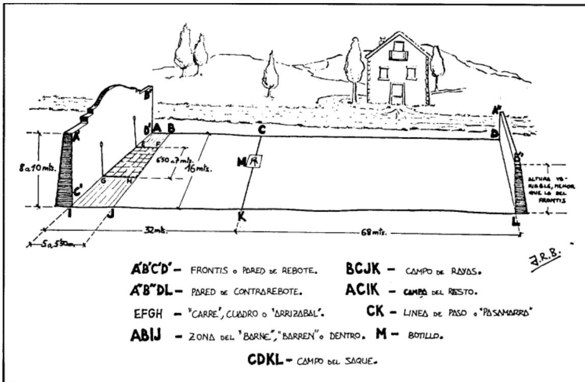
Frontón de rebote, según José R. de Basterra
