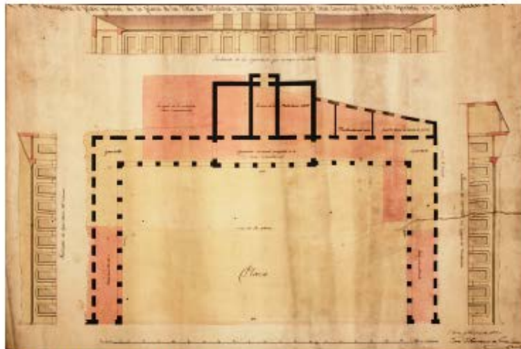
1850. Proyecto de Plaza y Casa Consistorial. Arquitecto José Eleuterio de Escoriaza (AM VILLABONA sin clasificación)
